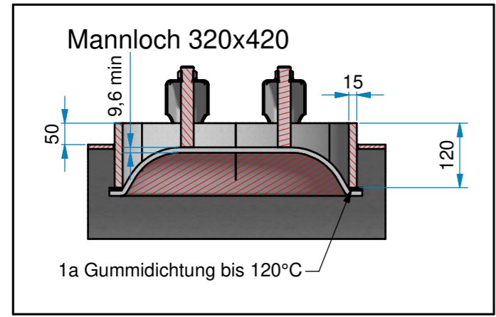
A-A (1:10)
